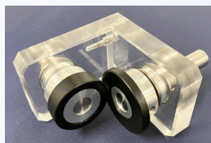
磁力锥齿轮
