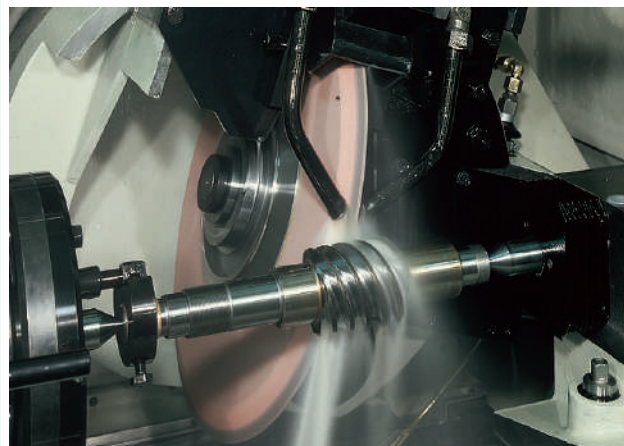
特别定制的蜗杆磨削机
