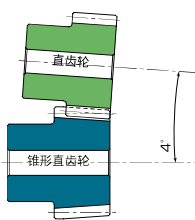
锥形直齿轮和普通直齿轮组合安装，则轴角为 4°。
