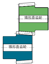
反向安装轮毂，则轴角变为 0° (平行轴)。
